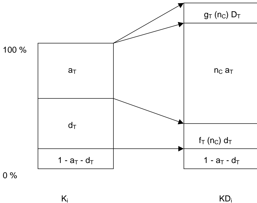
Abb. 5: Kosten einer Software-Entwicklungshase Testen bei einfacher Erstellung und bei n_C -facher Diversität
