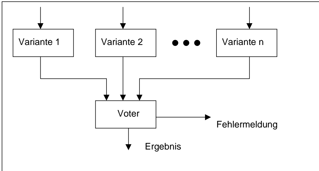
Abb. 2: Struktur der N-Varianten-Programmierung
